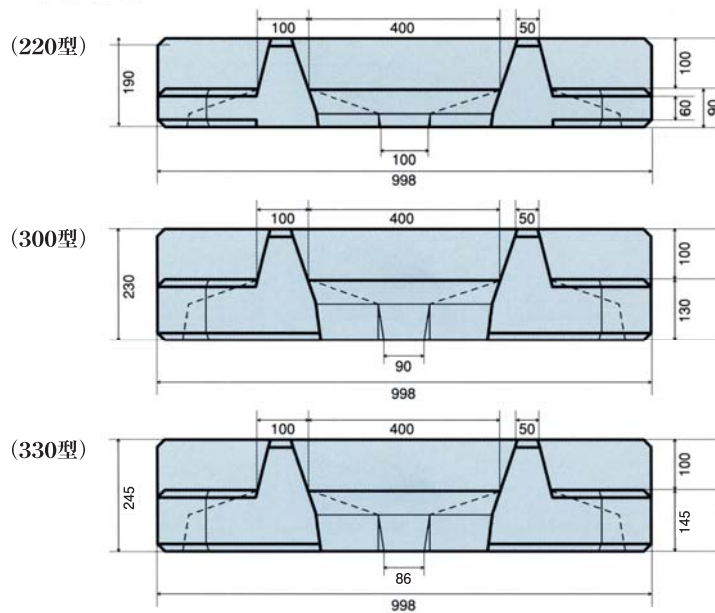
■ 展開平面図
