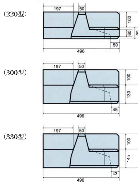
■ 1/2 側面図
