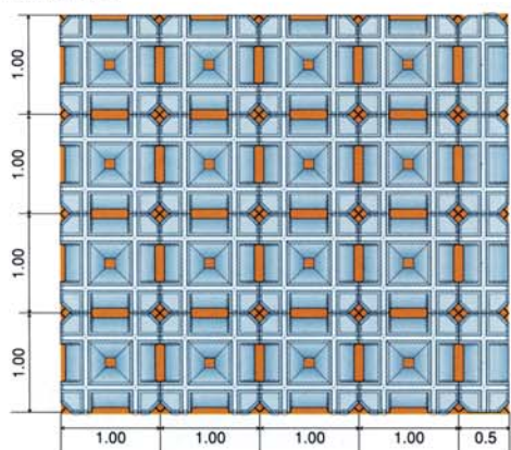
■ 展開平面図
