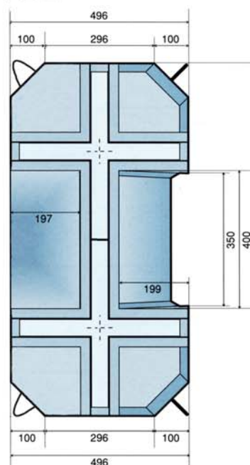
■ 1/2 側面図
