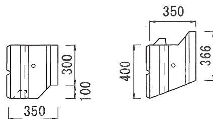
〔岩着型〕
