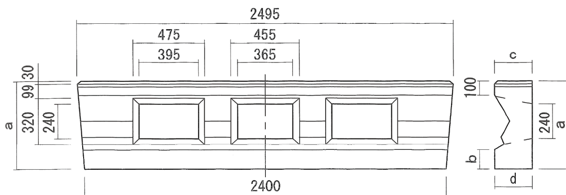
断面図
