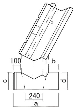
断面図
