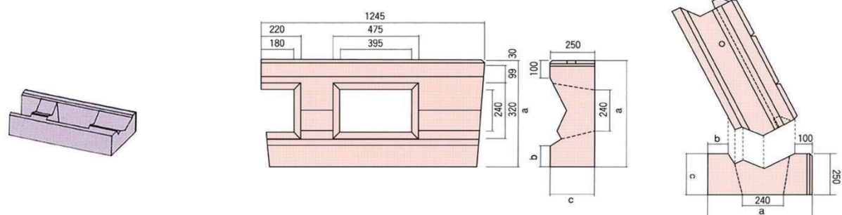
諸元表（5分勾配）
