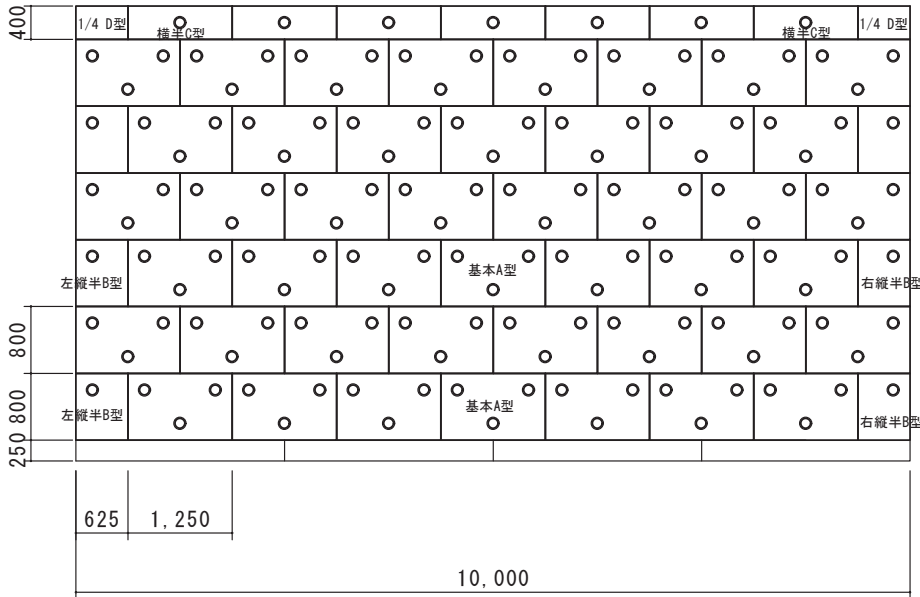
夢Ⅱ45型展開図
