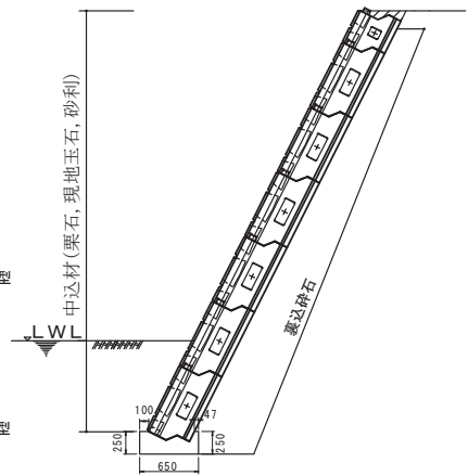
夢Ⅱ45型断面図
