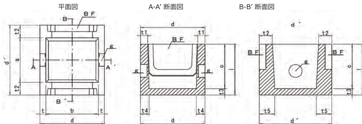
規格形状図
