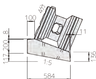
4分用路側基礎
