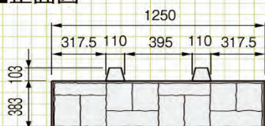
■正面図
