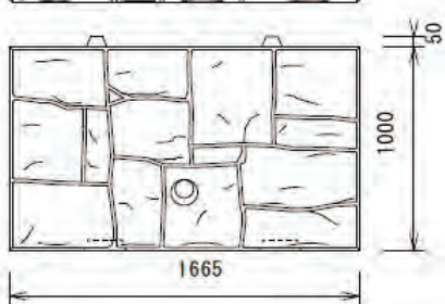
正面図
