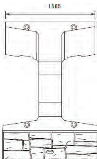
上面図
