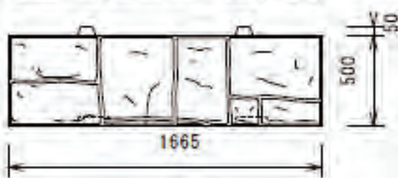
正面図
