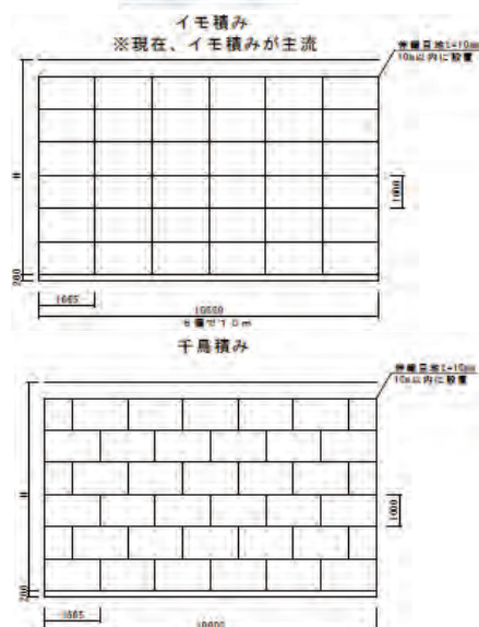
標準展開図
