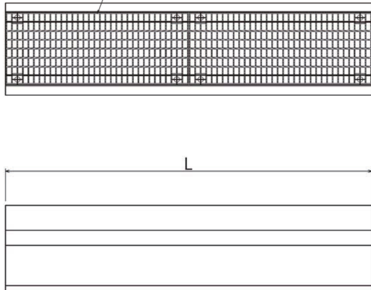
グレーチング（4点固定）
