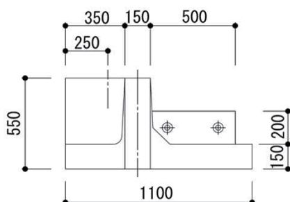
断面図（A-A）
