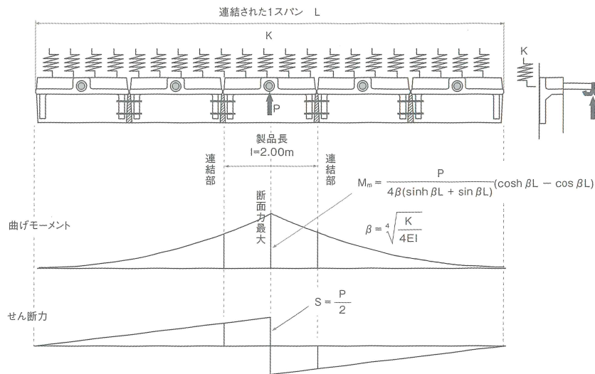
縦方向に発生する曲げモーメントとせん断力図
