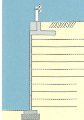
補強土壁
