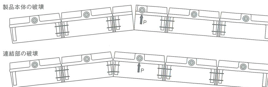
図-2 プレガードの縦方向の破壊形態
