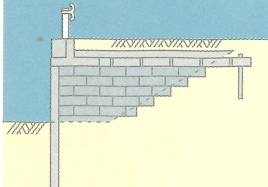
軽量盛土
