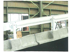
縦断16%の設置確認
